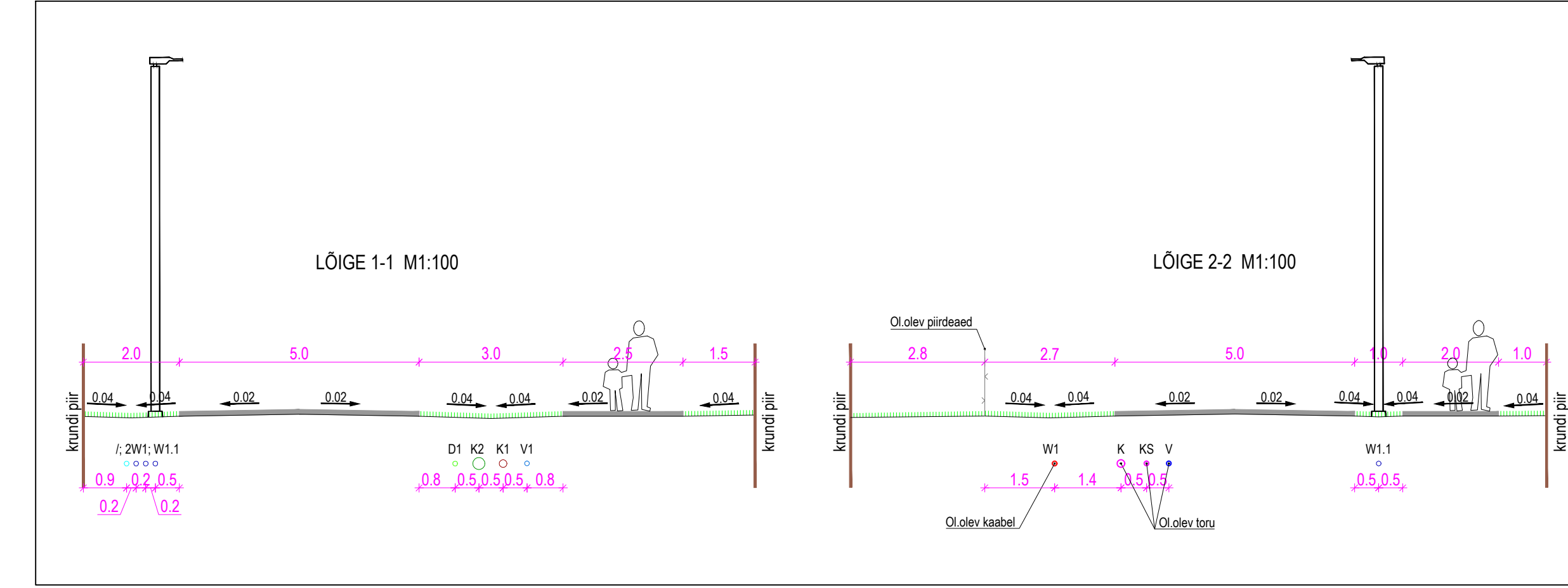
Joonis 5.4 LÕIKED
