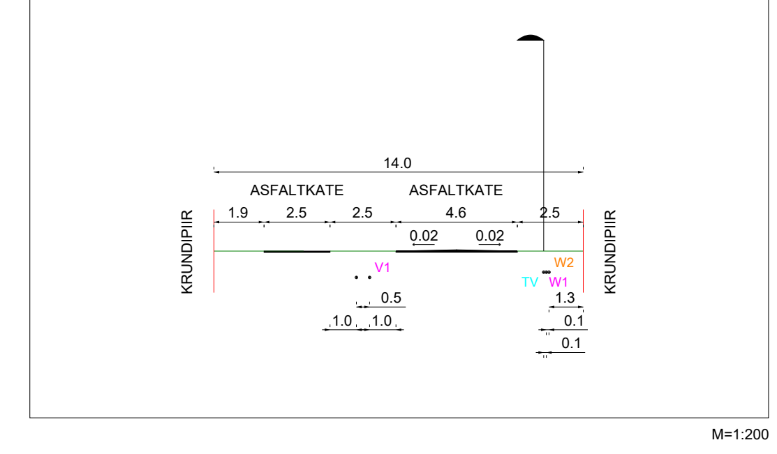
TÄNAVA RISTLÕIGE. LÕIGE C - C
