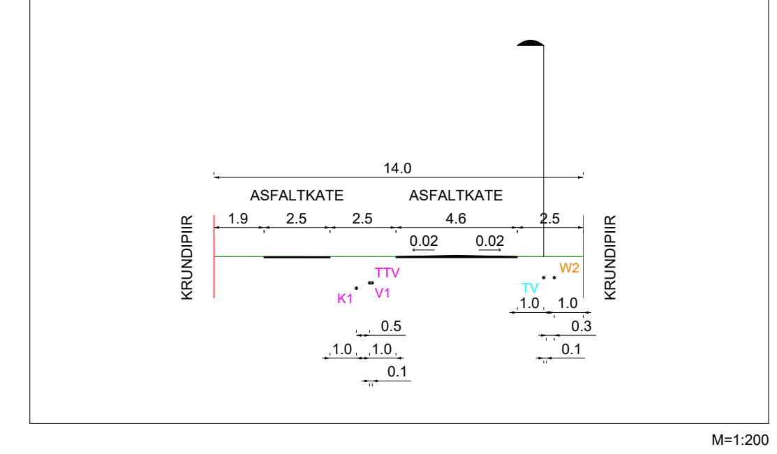
TÄNAVA RISTLÕIGE. LÕIGE B - B
