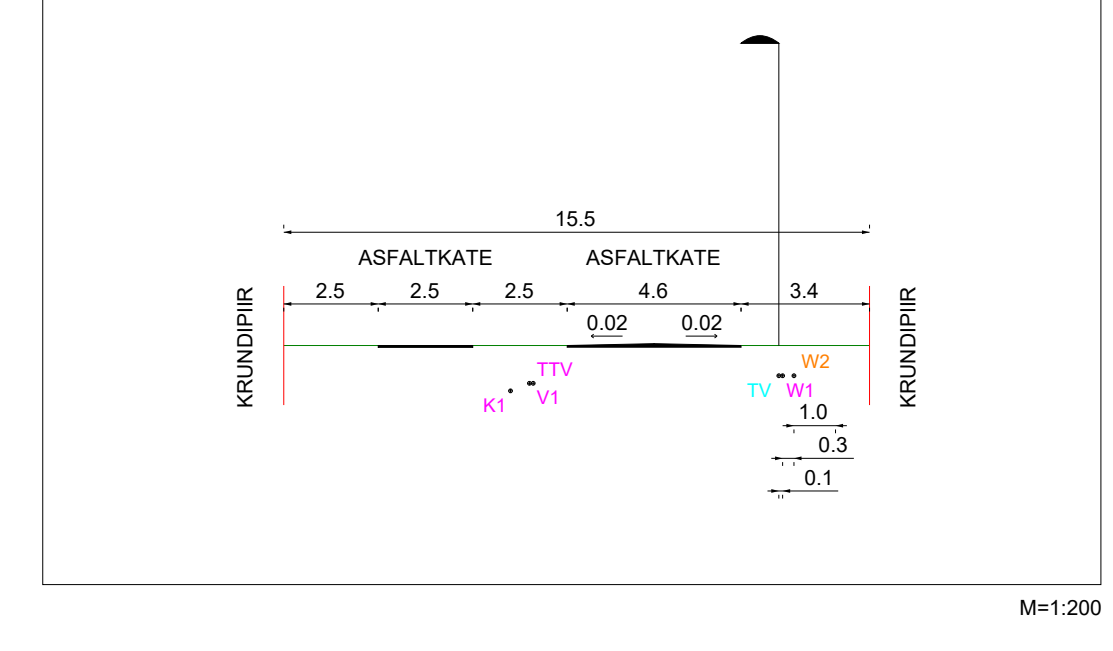
TÄNAVA RISTLÕIGE. LÕIGE D - D
