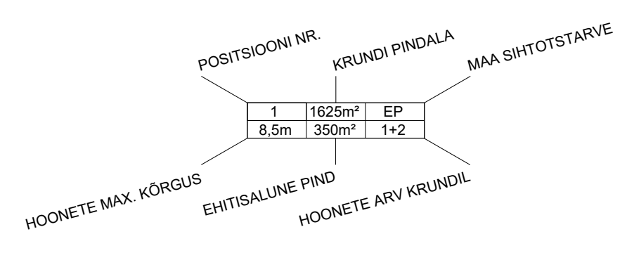
TÄNAVA RISTLÕIGE. LÕIGE A - A
