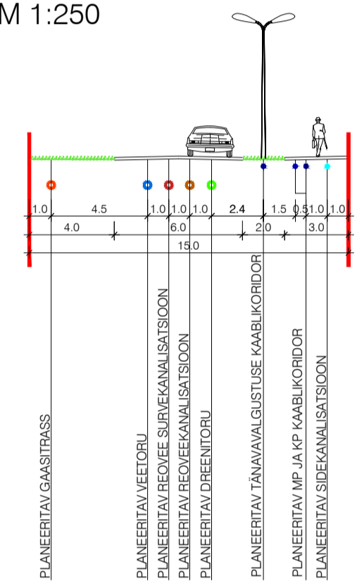
TÄNAVA RISTLÕIGE 1-1 M 1:250
