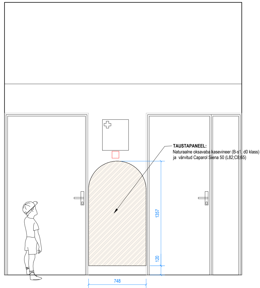
PANEEL 7.2A
