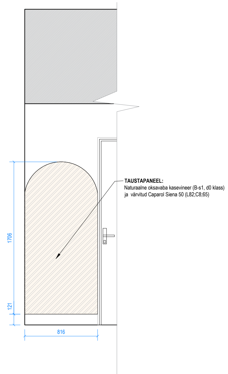
PANEEL 7.2B
